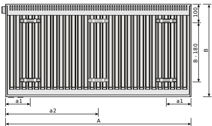
Ventil Compact / Plan Ventil Compact Typ 11, Rückansicht
